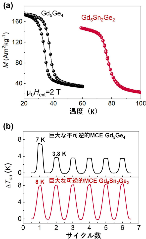
図 2. \text{Gd}_5\text{Sn}_2\text{Ge}_2 化合物における高効率な磁気熱量効果 (MCE)。(a) 2T の磁場下における磁化 ( M ) の温度変化。曲線が開いた部分の面積がエネルギー損失に対応する。(b) \text{Gd}_5\text{Ge}_4 化合物の断熱温度変化 ( \Delta T_{ad} )。(b の上図) では、 \Delta T_{ad} に巨大な MCE が観測されますが、これは反復磁場下では維持されません。これに対し、 \text{Gd}_5\text{Sn}_2\text{Ge}_2 化合物 (b の下図) では、巨大かつ可逆的な MCE を実現しています。
