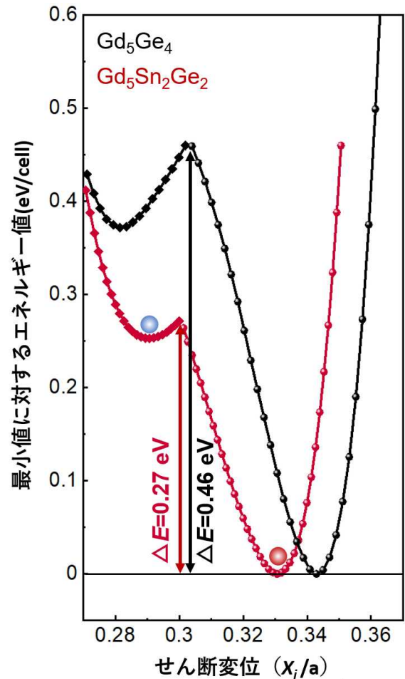
図 3. せん断変位を関数とする活性化障壁。 \text{Gd}_5\text{Sn}_2\text{Ge}_2 化合物の場合、青丸と赤丸はそれぞれ局所極小点と全極小点を示します。Sn 合金化後、相転移の活性化障壁 \Delta E は大幅に低減されます。
