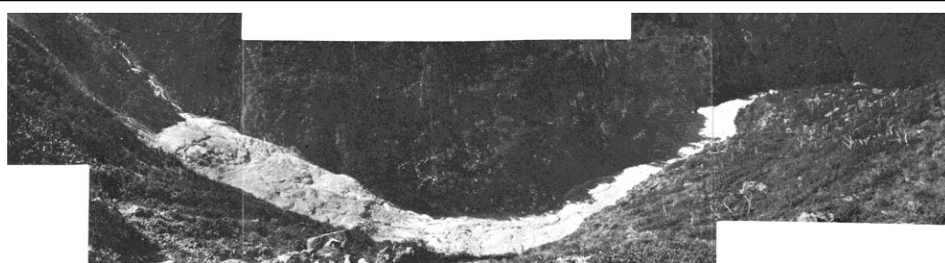
図1 1936年溶融硫黄噴火の際に硫黄で埋まったカムイワッカ川。渡辺・下斗米(1937)北海道地質調査会報告9より引用。
