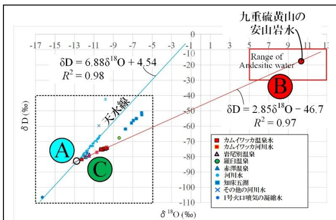
図3 知床硫黄山周辺で採取した水試料の水素・酸素同位体比のデルタダイアグラム。標準海水の水素・酸素同位体比(原点)を基準にして水素同位体比( \delta D )と酸素同位体比( \delta^{18}O )がどれくらい高いか低いを示します。水色の線はこの地域の降水の同位体比を表す天水線です。赤線は、カムイワッカ温泉水の同位体比の近似線。
