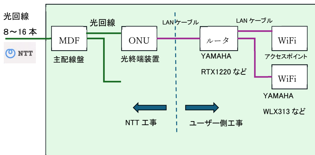
図6.1 臨時敷設工事の構成図
