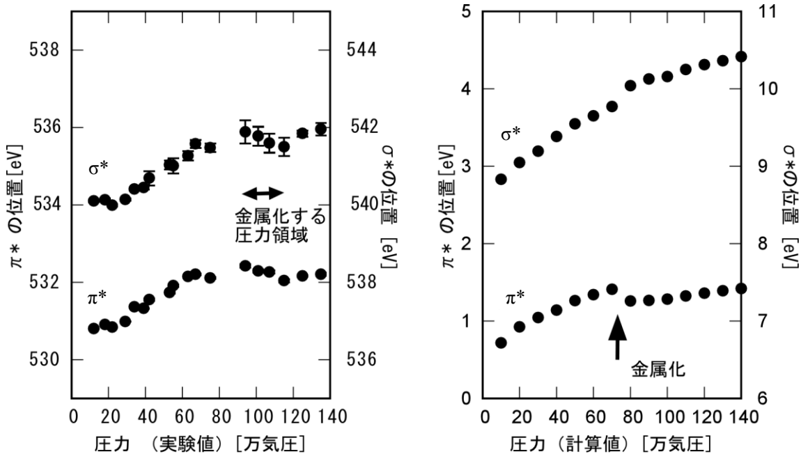
図 3. \pi^* バンドと \sigma^* バンドのエネルギーの圧力変化。金属化する前は加圧により高いエネルギーへとシフトしたが、金属化するには低いエネルギー側にシフトする（左）。金属化が終了すると、加圧により再び高いエネルギーへとシフトする。金属化に伴う \pi^* バンドの低エネルギーシフトは理論計算でも確かめられた（右）。
