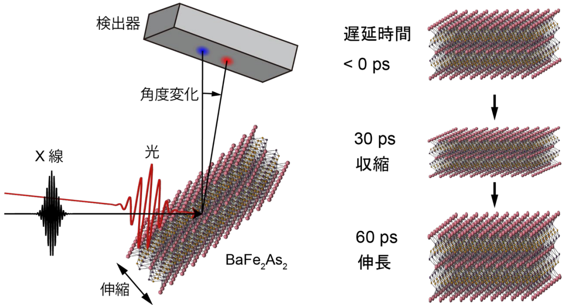
図1 時間分解 X 線回折法 の概念図 (左) と観測された結晶構造変化 (右)
