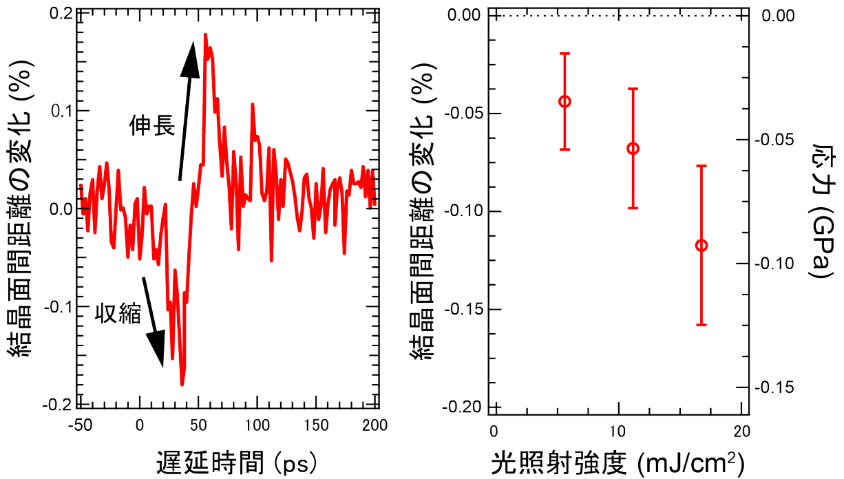
図2 結晶面間距離の時間依存性 (左) と収縮の光照射強度依存性 (右)。(左) 図の遅延時間では光照射した時間をゼロとする。
