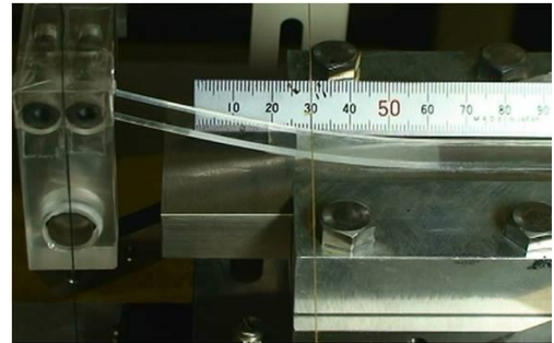
皮膜の引き剥がし試験
