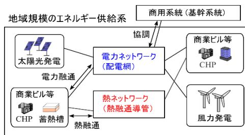
地域規模のエネルギーシステム概念図
