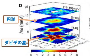
\alpha RuCl 3 非弾性中性子散乱実験
