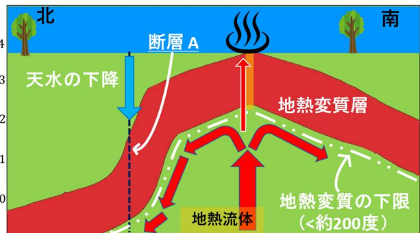
熱水循環の概念図
