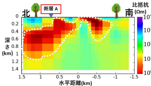
地熱地域の地下比抵抗構造（南北断面）
