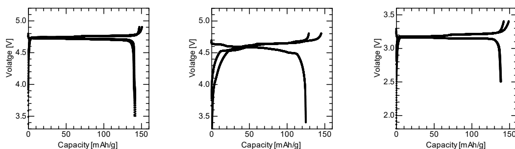
図 1. 金属リチウム負極, MCMB グラファイト負極, \text{Li}_4\text{Ti}_5\text{O}_{12} 負極と組み合わせた二次電池の初期充放電曲線
